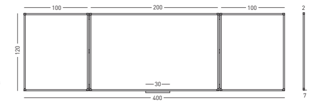
720/T2 120 x 400 120 x 200 2 + 4 30
